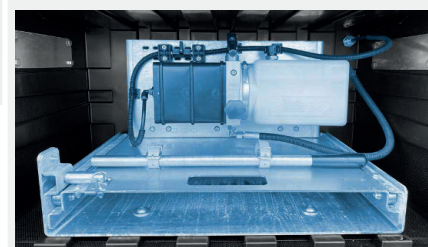
Pompe hydraulique pour réhausser la carrosserie
