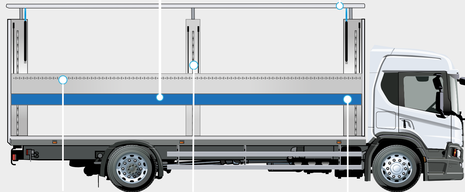
Seitenbordwände mit integrierten Ladungssicherungsschienen
