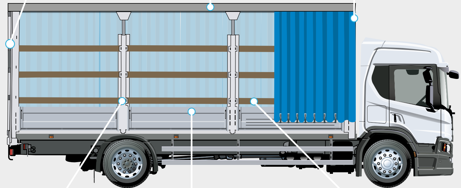
Seitenbordwände mit je nach Aufbauhöhe nötigen Planenfixier- profilen
